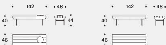
Panchetta con e senza ripiano / Bench with and without shelf
